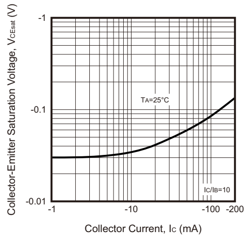
Fig.3 - V_{CEsat} - I_C
